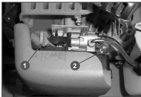
Рис. 12 Ручной топливный насос и рычаг управления воздушной заслонкой
