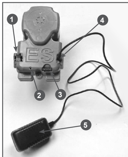
Рис. 21 Зарядка аккумулятора
