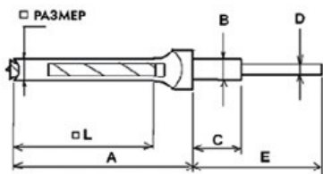
РАЗМЕРЫ ДОЛБЕЖНЫХ РЕЗЦОВ И СВЁРЛ JET
