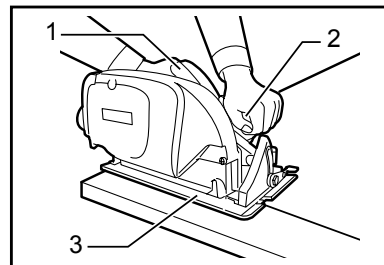
1. Poignée arrière 2. Poignée avant 3. Base
