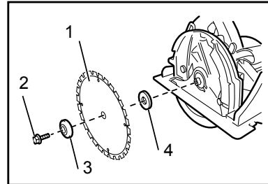
1. Lame 2. Boulon hexagonal 3. Bague externe 4. Flasque intérieur
