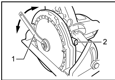
1. Clé 2. Verrouillage de l'arbre
