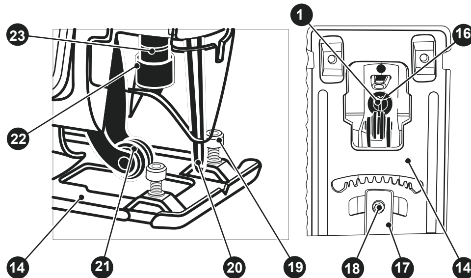
Рисунок А — общий вид лобзика.
