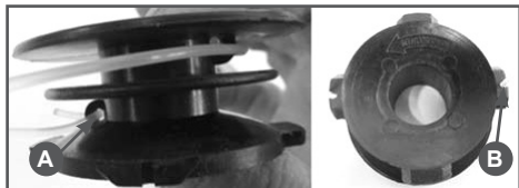
Рис.14 Установка корда
