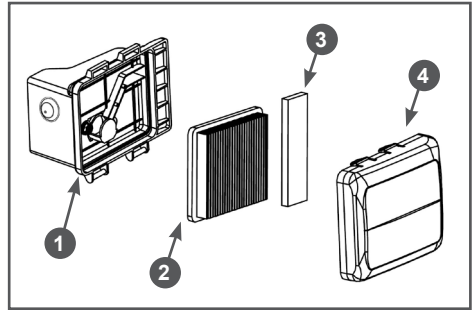
Рис. 18 Обслуживание воздушного фильтра
