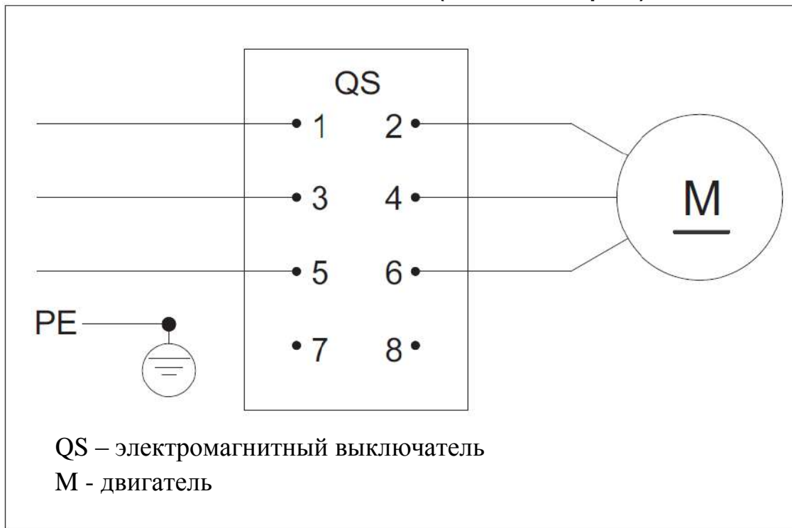
Схема подключения для DS150/DS250 (230В/50Гц/1 фаза)
