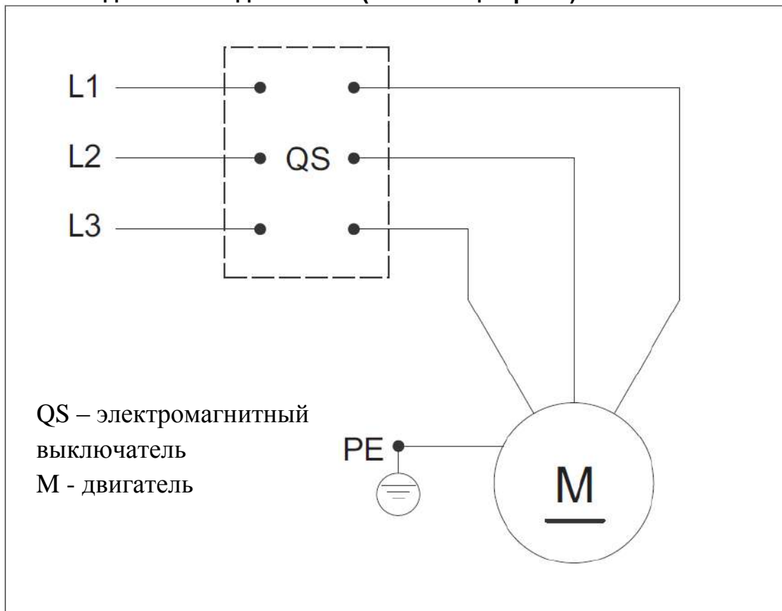
Схема подключения для DS250 (380В/50Гц/3 фазы)
