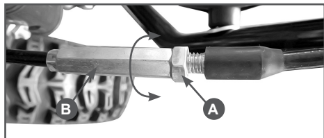
Рис.14 Регулировка троса привода шнека
