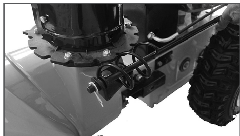
Рис. 6 Установка нижней части рычага поворота желоба
