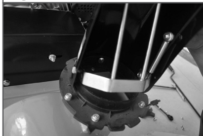
Рис. 5 Установка разгрузочного желоба
