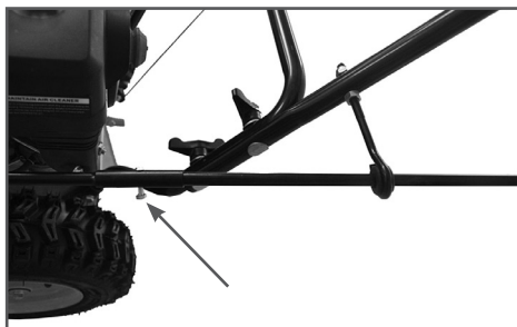
Рис. 8 Соединение верхней и нижней половины рычага поворота желоба
