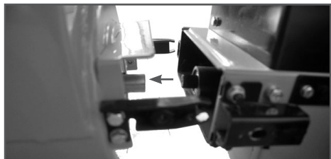
Рис. 3 Центровка валов отбора мощности машины и снегоотбрасывателя
