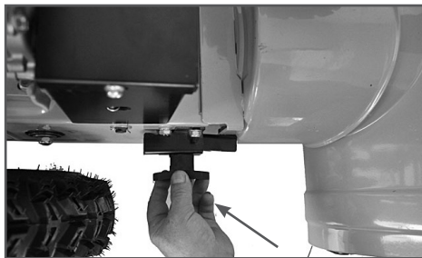
Рис. 4 Закрепление снегоотбрасывателя
