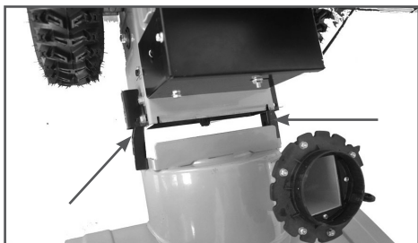
Рис. 2 Стыковка снегоотбрасывателя
