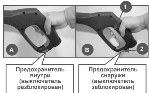
Рис. 7 Предохранитель выключателя пистолета
